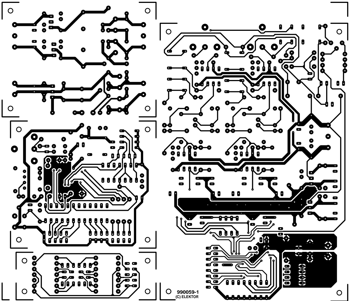
soldeerzijde
