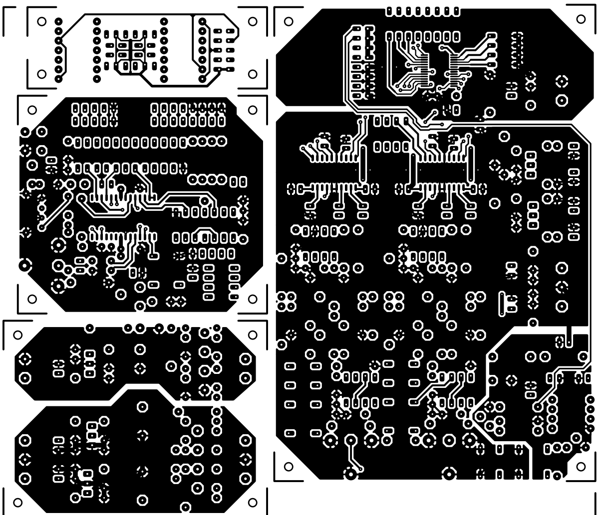
componentenzijde
