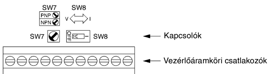
PNP jelleg
