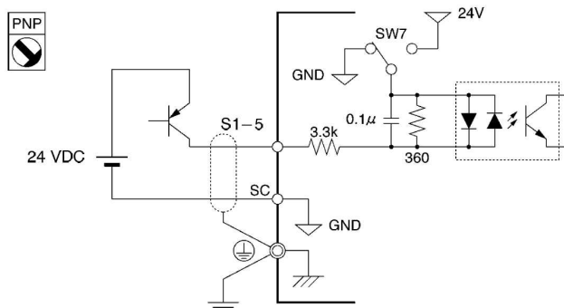
PNP jelleg
